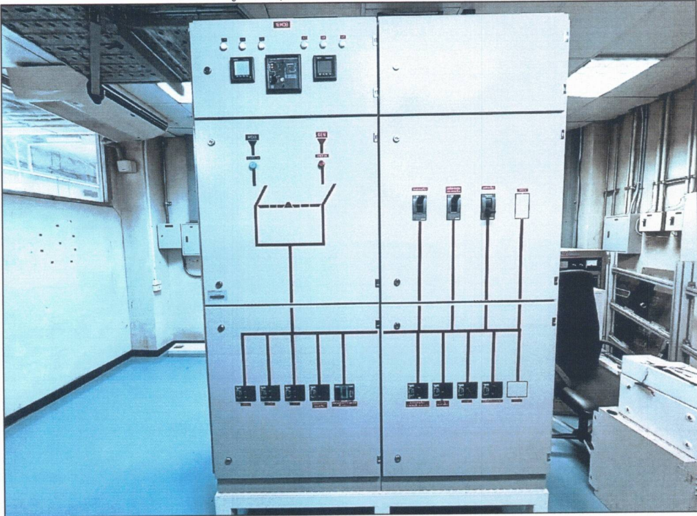
ตู้ไฟฟ้าสำรอง (EMDB)
